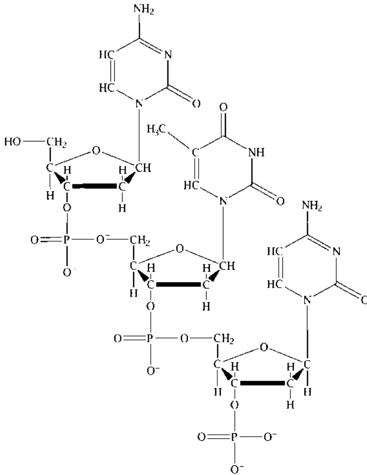
شكل ٢-٥: قطاع من تركيب الدي. إن. إيه. يوضح الروابط التي تحدث بين النيكليوتيدات.
