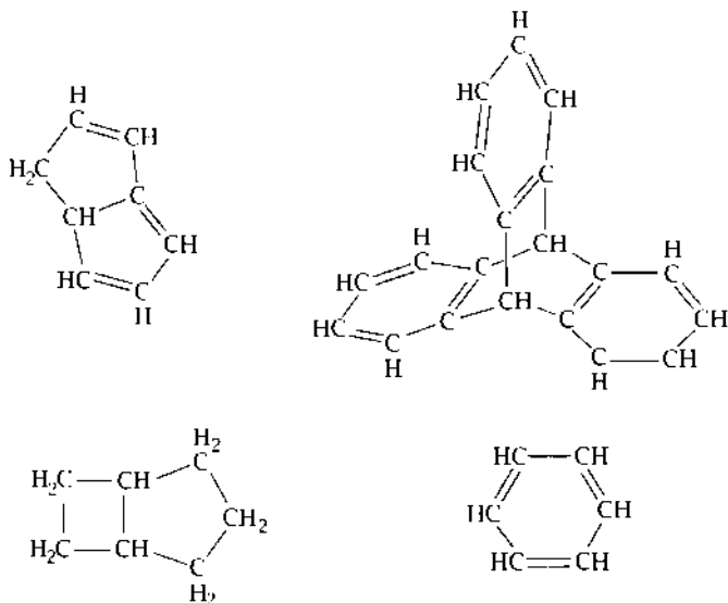
شكل ٢-١-٥: بعض تركيبات الهيدروكربونات ذات الحلقات.
