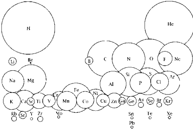
شكل ١-٢-٧: انتشار العناصر الموجودة في الشمس. عُذلت بناء على تصريح من ستيفن أي. داتش لمقال «الجدول الدوري للعناصر المنتشرة» الصادر عن مجلة تعليم الكيمياء عدد ٧٦ (١٩٩٩): صفحة ٥٨-٣٥٦.
