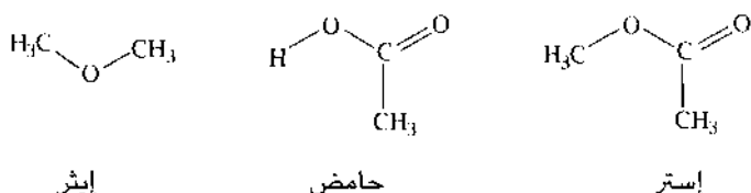
شكل ١-٢-٧: مثالاً على الإيثر والحامض والإستر.
