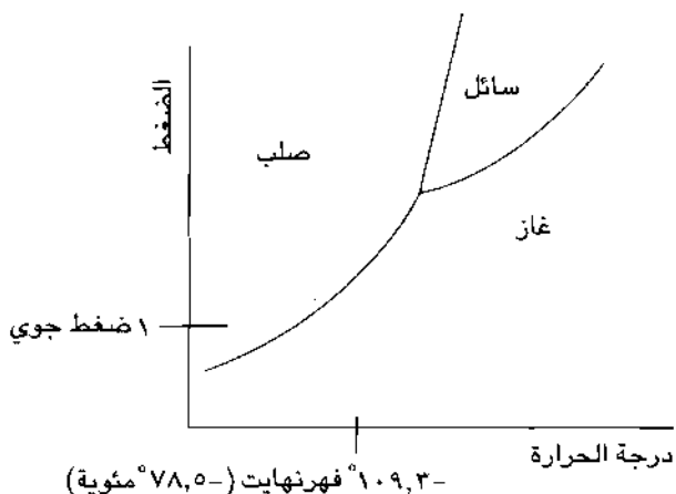
شكل ١-١٤-٣: مخطط الطور لثاني أكسيد الكربون.
