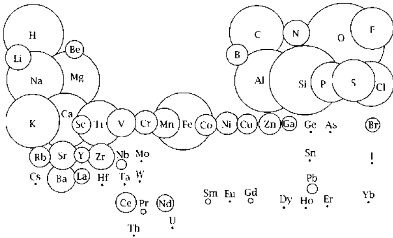
شكل ٨-٢-١: انتشار العناصر في قشرة الأرض. وقد عُدلت بناء على تصريح من ستيفين أي. داتش عن مجلة تعليم الكيمياء «الجدول الدوري للعناصر الغزيرة» ٧٦ (١٩٩٩): ٥٨-٣٥٦.
