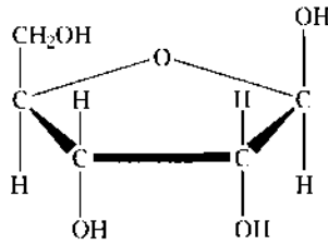
شكل ٢-١-٣: السكريد: وحدة بناء الكربوهيدرات.
