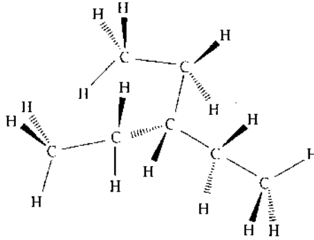
شكل ٣-١-٢: سلسلة مكونة من سبع ذرات كربون ملفوفة حول روابطها.
