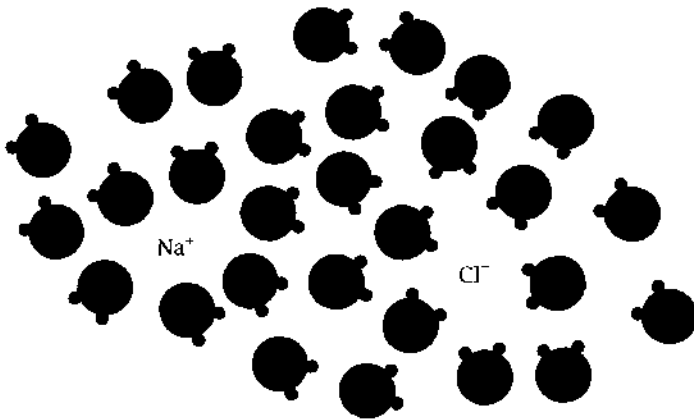
شكل ١-٥-٢: جزيئات الماء التي تعزل أيون الصوديوم وأيون الكلور عن طريق تكوين أقفاص المذيب حول الأيونات.
