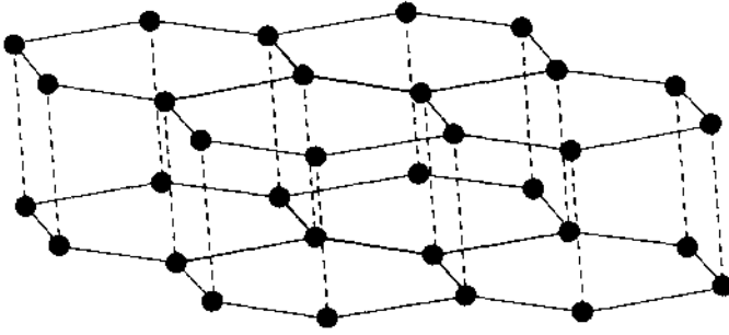
شكل ١-١٢-٤: الجرافيت هو كربون مرتبط تساهميًا في شكل أفخر سداسية.
