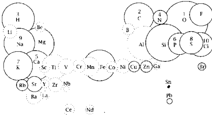
شكل ١-٢-٩: مقارنة بين عناصر القمة الأربعين الموجودة في القشرة الأرضية وعناصر القمة العشرة في جسم الإنسان، وتُرقم العناصر الموجودة في الجسم لبيان انتشارها، ويكون الأوكسجين المرقم برقم (١) أكثرها وفرة، ثم يليه الكربون المرقم برقم (٢)، إلخ.
